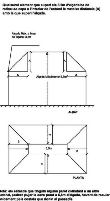
EXEMPLE DE RECLADA SEGONS ALÇADA
