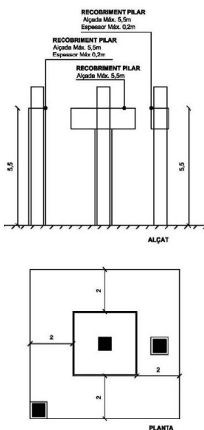
EXEMPLE DE RECOBRIMENT DE PILARS
