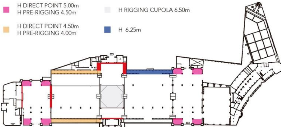
Alturas espaciales rigging / Special heights for rigging
